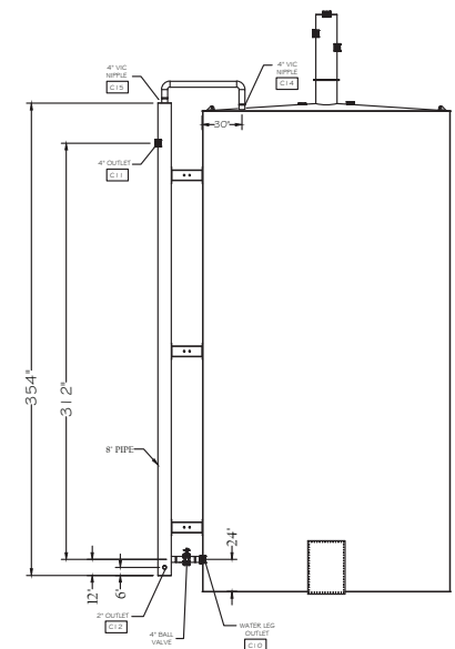
270° (WATERLEG DETAIL)
